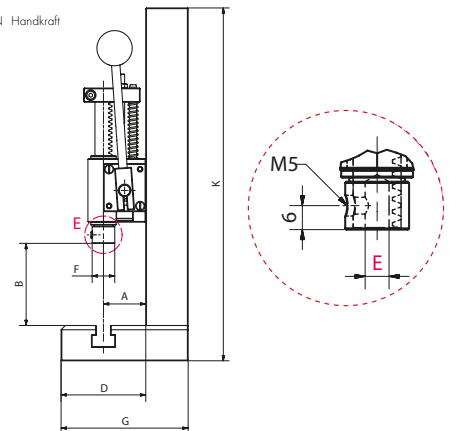
Zahnstangenpresse MPZ 500-30
